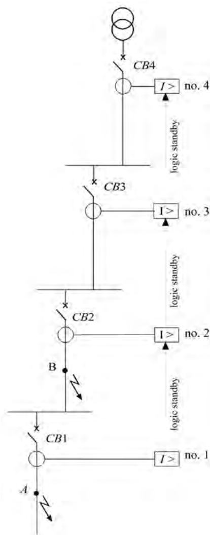
Figure II.3- Sélectivité logique
