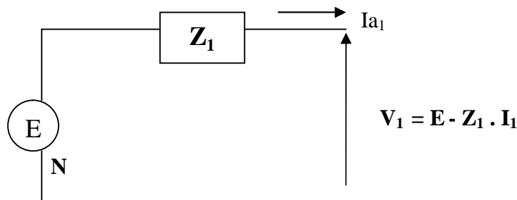
Figure 2 - Système direct d'une seule phase
