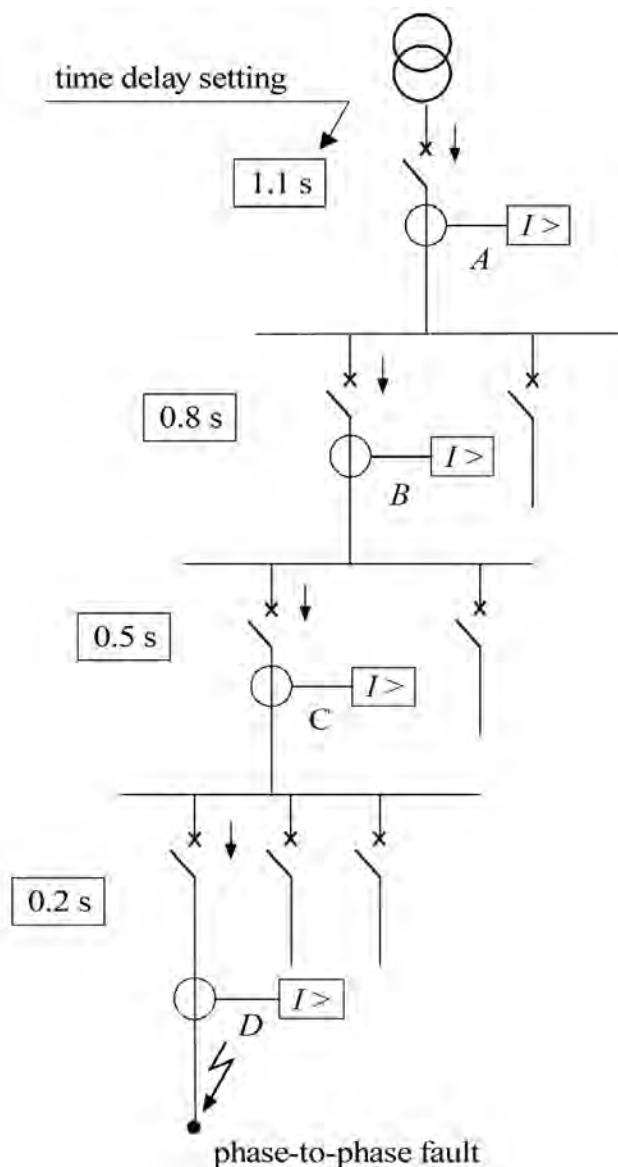
Figure II.2- Sélectivité temps-classé
