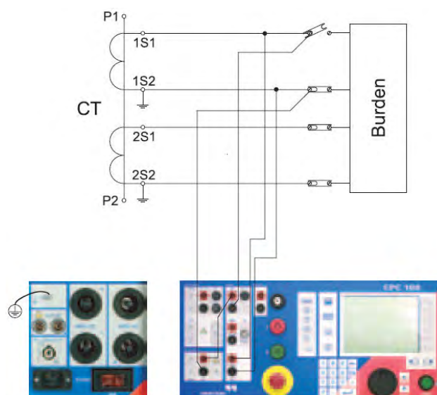
Figure III.4-Schéma de raccordement du CPC100 au TC
