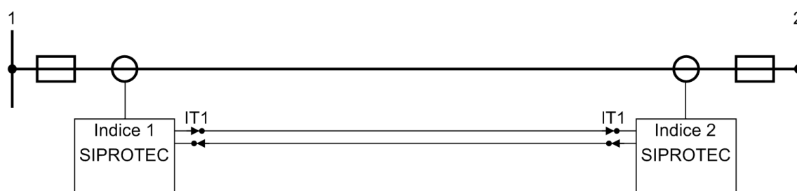
Figure IV.7- Système de protection de distance à deux extrémités comprenant deux relais dotés d'une interface de téléprotection chacune (émetteur/récepteur).
