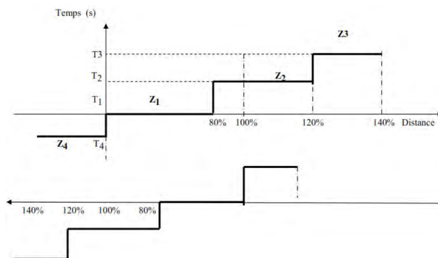
Figure IV.3- Sélectivité chronométrique de protection à distance
