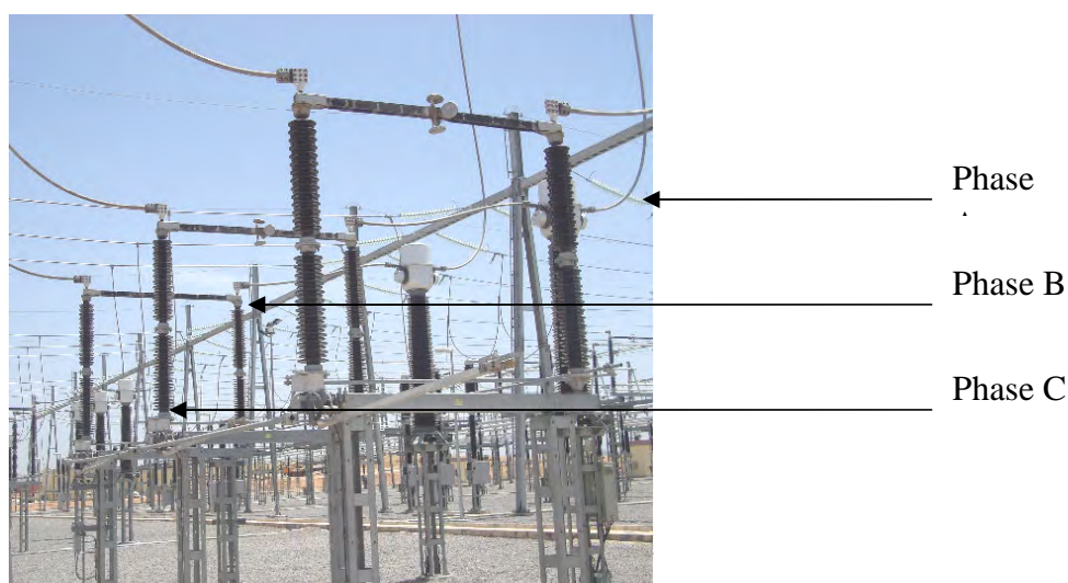
Figure I.12 - Sectionneur de ligne
