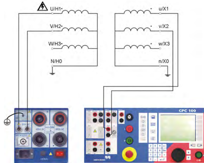
Figure III.13- Schéma de raccordement du CPC100 au TP
