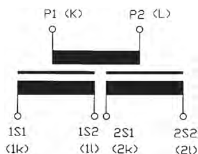
Figure III.2- Désignation des bornes du transformateur de courant
