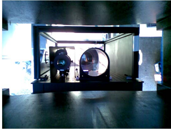
Fig III.7–Le système instrumentale Lidar LESAA, vue de haut.
