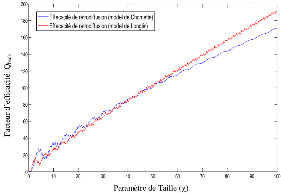
Fig IV.20 – Facteurs d'efficacités de rétrodiffusion Q_{back} en fonction de paramètre de taille \chi , pour les deux modèles Longtin et Chomette à 550nm
