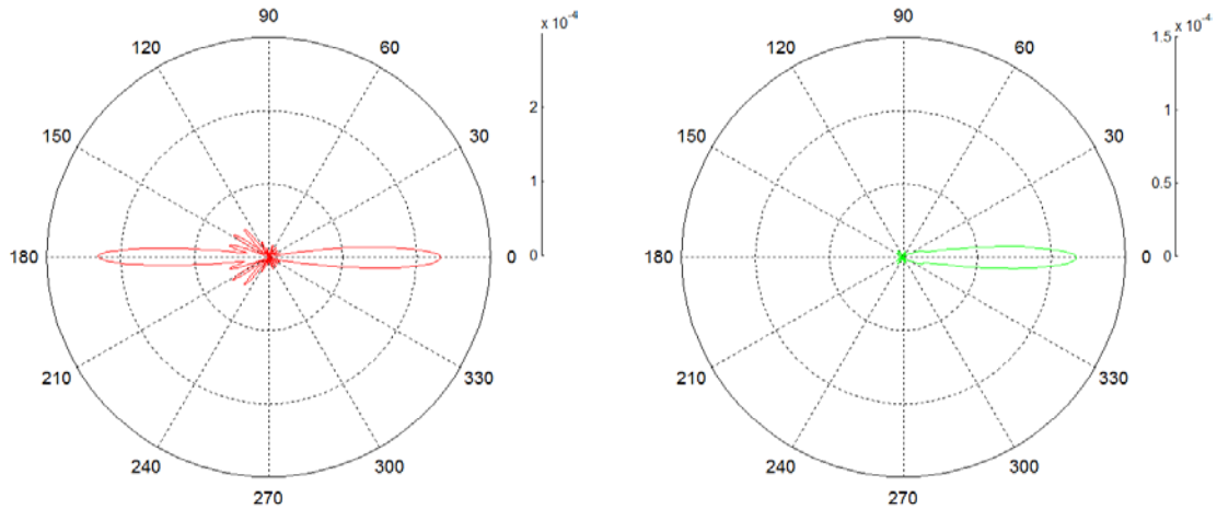
Fig IV.24 Indicatrices de diffusion normalisée simulées par un code de Mie à \lambda=550 \text{ nm} et \chi=10 pour différents types de particules (a : particule désertique selon le modèle de Chomette, b : composante carbonée, c : composante hydrosoluble, d : quartz + 10% hématite)
