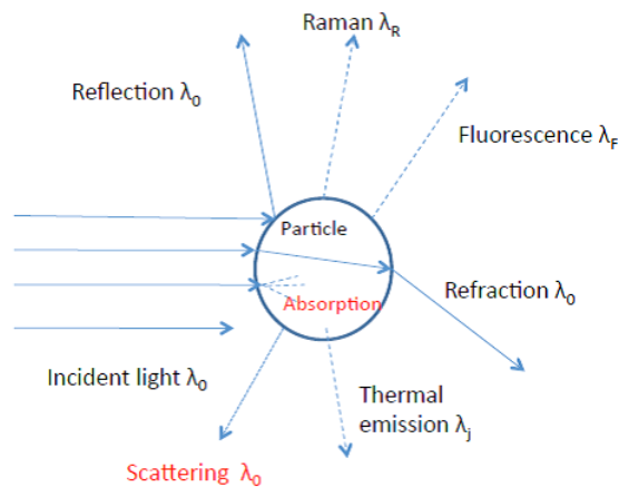
Fig III.4– Interaction lumière-particule [J. H. Seinfeld, S. N. Pandis, 1998]
