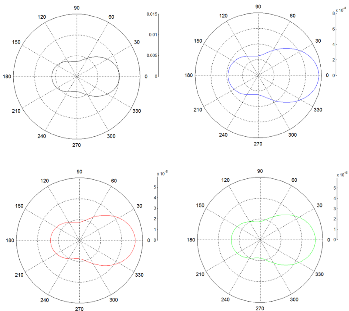
Fig IV.21 Indicatrices de diffusion normalisée simulées par un code de Mie à \lambda=550 nm et \chi=0.1 pour différents types de particules (a : particule désertique selon le modèle de Chomette, b : composante carbonée, c : composante hydrosoluble, d : quartz + 10% hématite)
