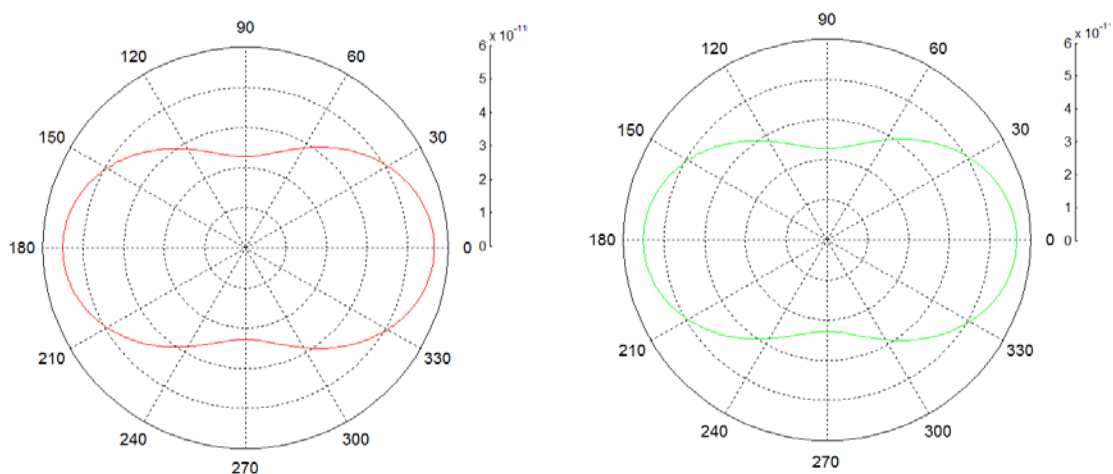
Fig IV.21 Indicatrices de diffusion normalisée simulées par un code de Mie à \lambda=550 nm et \chi=0.1 pour différents types de particules (a : particule désertique selon le modèle de Chomette, b : composante carbonée, c : composante hydrosoluble, d : quartz + 10% hématite)
