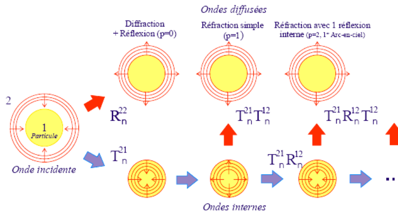
Fig II.16 – schéma d'interprétation de la méthode de décomposition de Debye [Hovenac E, 1992]
