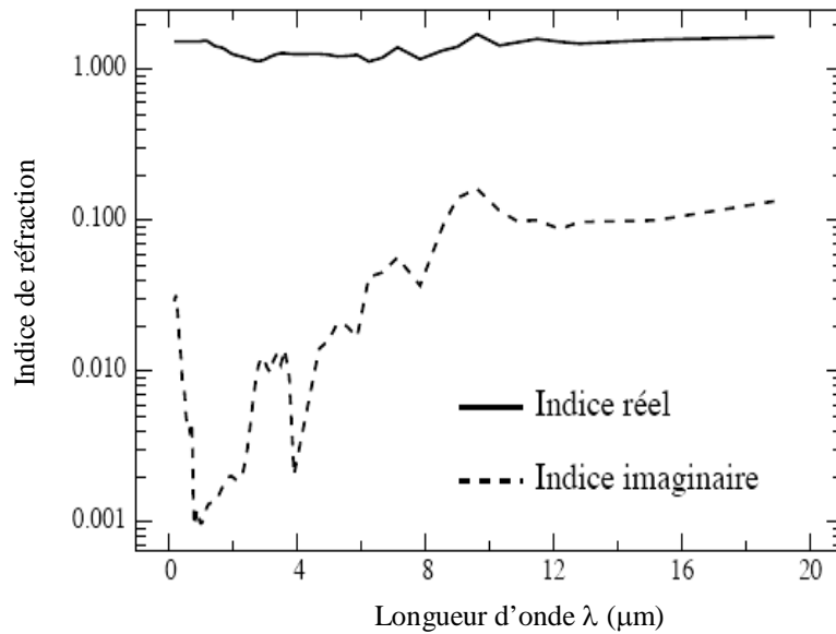
Fig IV.14– Indices complexes de réfraction utilisés dans la modélisation de Chomette.
