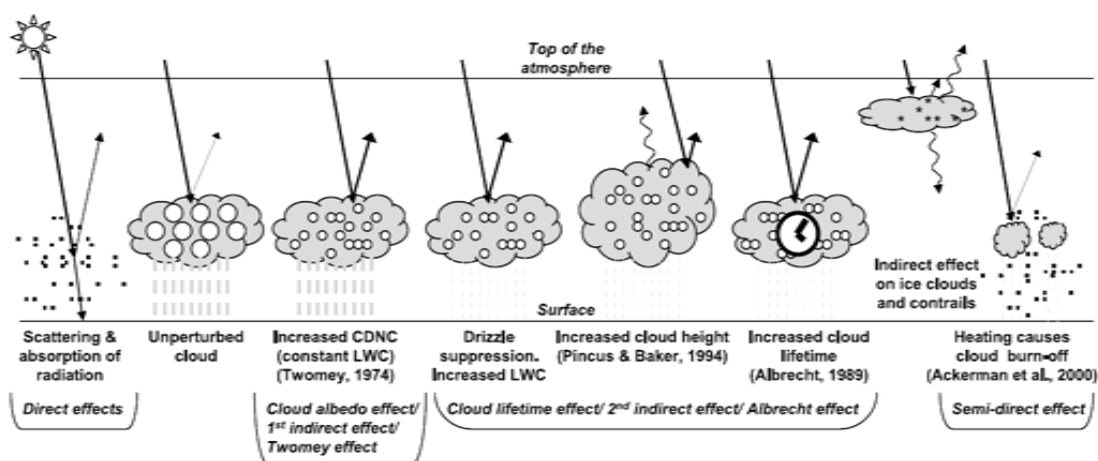
Fig I.14–Représentation de différents mécanismes radiatifs associés aux effets des nuages en liaison avec les d’aérosols [Haywood and Boucher, 2000]
