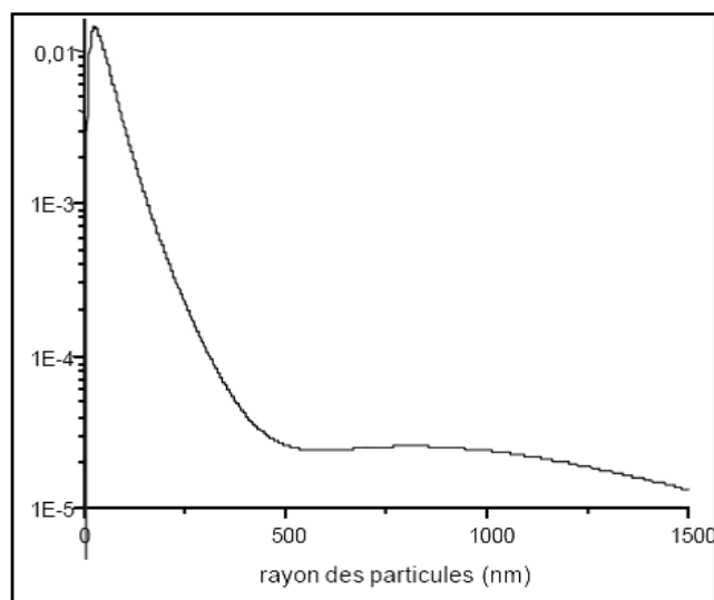
Fig IV.2 – Distribution de taille normalisée des aérosols urbains effectuée dans le cadre de la campagne, estimée à partir de l'étude par MEB des filtres impactés
