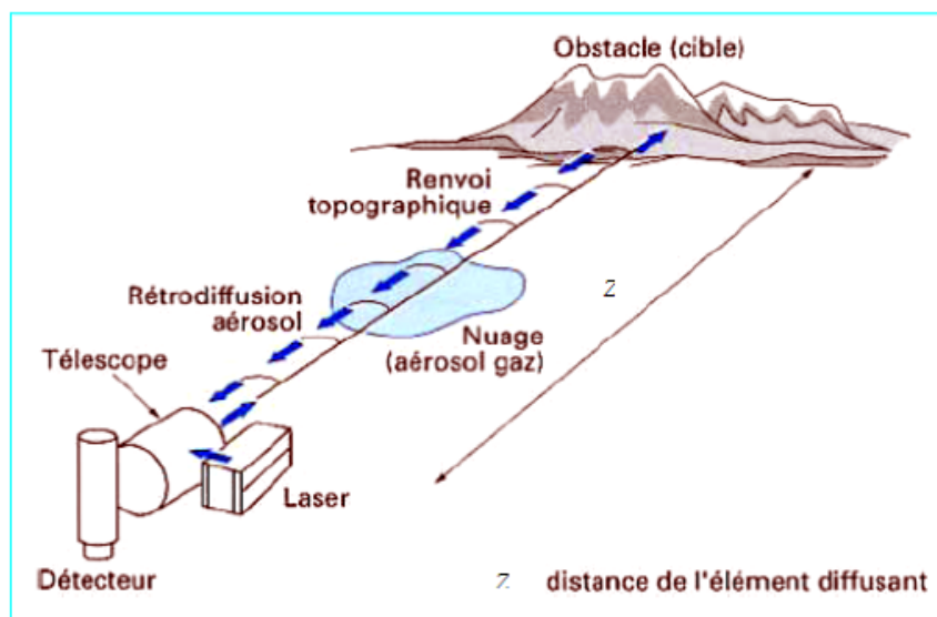
Fig III.2– Principe du Lidar atmosphérique
