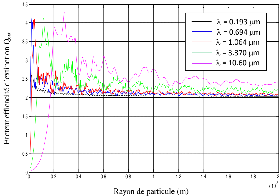
Fig IV.25 – Facteurs d'efficacités d'extinction de Mie, calculés en fonction de rayons de particule et à plusieurs longueurs d'onde en utilisant le modèle de Longtin
