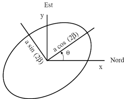
Fig. II.5 – Paramètres décrivant une onde simple polarisée elliptiquement.
