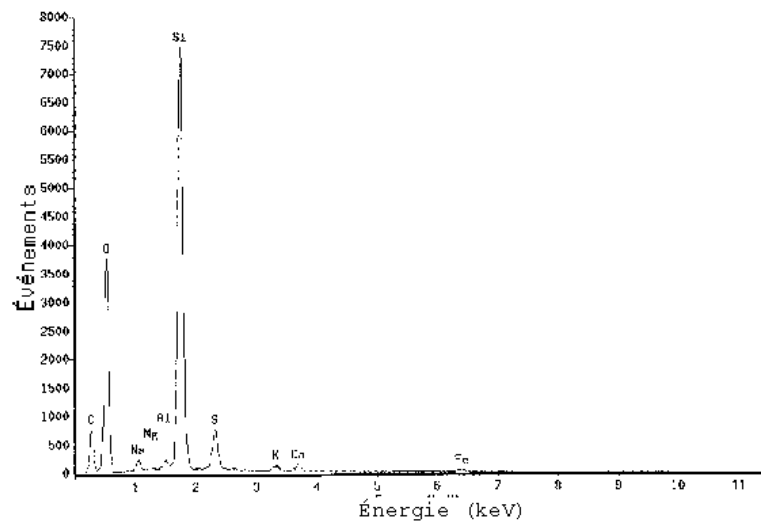
Fig IV.4 – Spectre de microanalyse d'une zone de filtre correspondant à une particule lisse de 1 µm de diamètre
