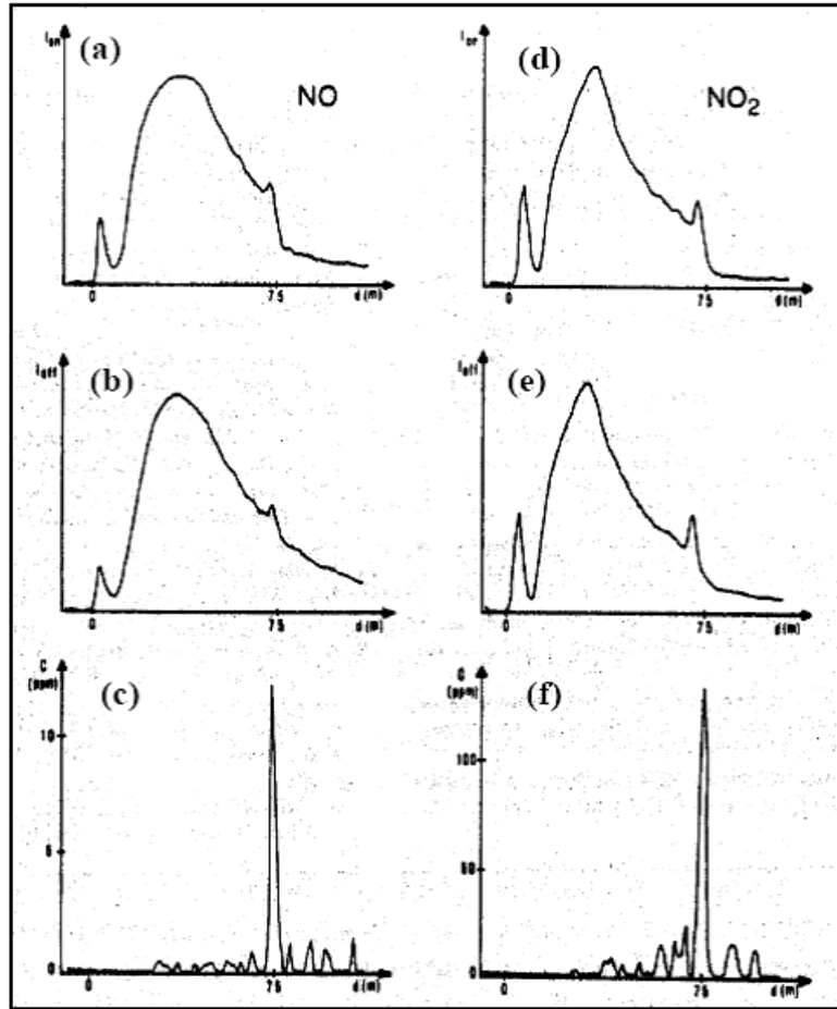
Fig III.16 – Exemples de mesures de concentrations [Kölsch H. J., Rairoux P., et al 1989] pour NO (c) et NO 2 (f) par méthode DIAL à partir des mesures de \lambda_{ON} ((a) et (d)) et \lambda_{OFF} ((b) et (e)).
