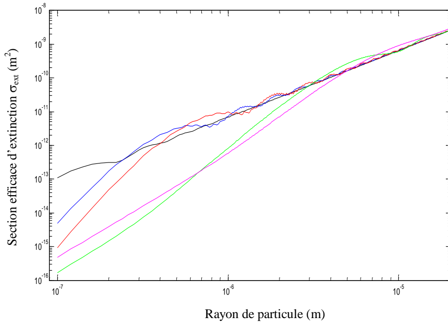
Fig IV.30 – Sections efficaces d'extinction de Mie, calculées en fonction de rayons de particule et à plusieurs longueurs d'onde en utilisant le modèle de Chomette
