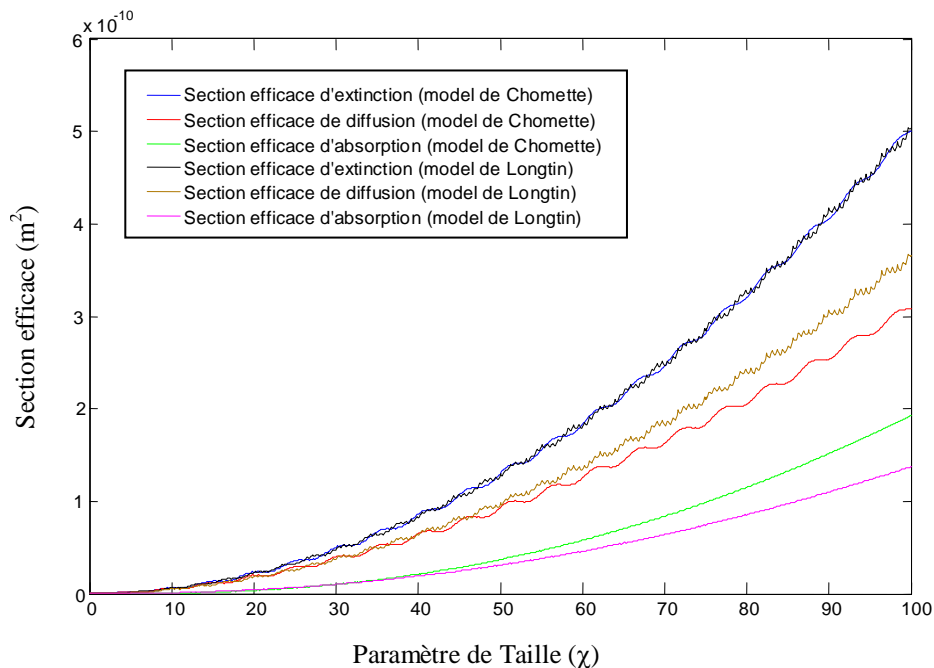
Fig IV.17 – Sections efficaces d'extinction \alpha_{ext} , de diffusion \alpha_s et d'absorption \alpha_{abs} en fonction de paramètre de taille \chi , pour les deux modèles Longtin et Chomette à 550nm
