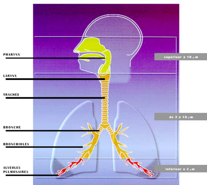
Fig I.13 – Appareil respiratoire et pénétration des particules [CITEPA, 2001]
