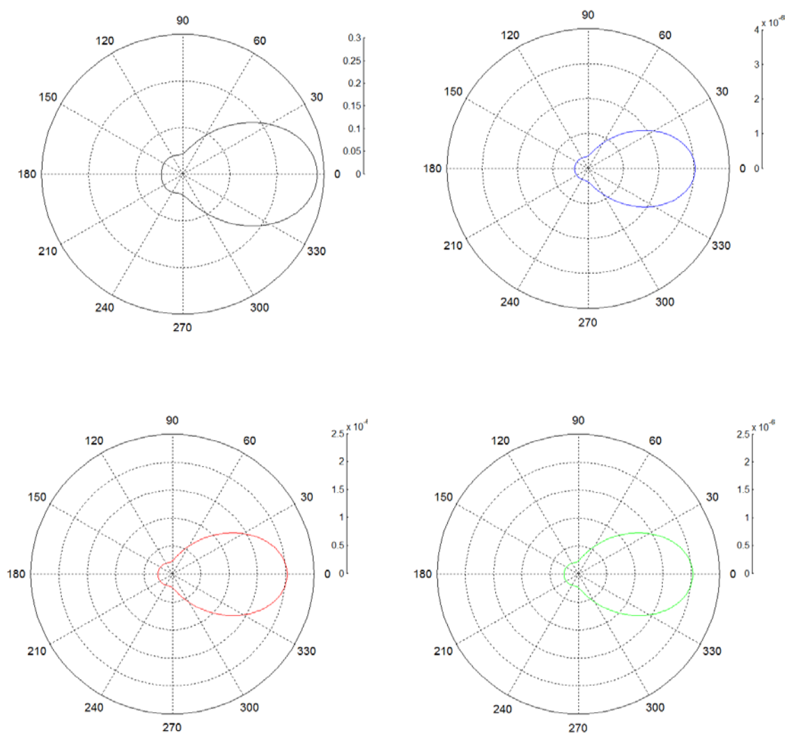
Fig IV.23 Indicatrices de diffusion normalisée simulées par un code de Mie à \lambda=550 nm et \chi=1 pour différents types de particules (a : particule désertique selon le modèle de Chomette, b : composante carbonée, c : composante hydrosoluble, d : quartz + 10% hématite)
