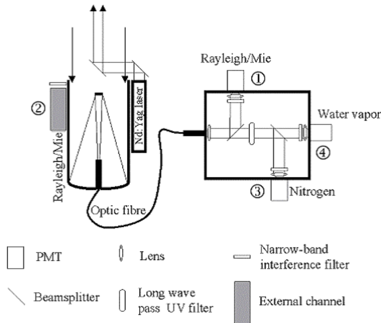
Fig III.17–Vue schématique du Lidar Raman IGN-SA. Les voies d'acquisition sont numérotées de 1 à 4.
